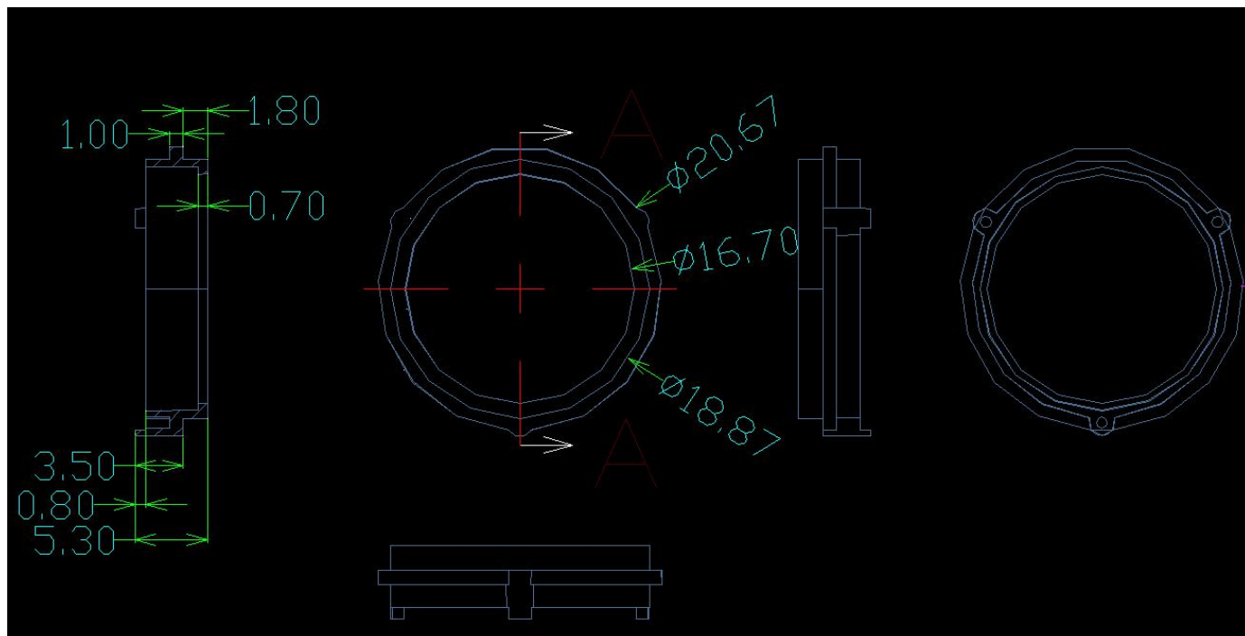
图2-1 A20尺寸图
