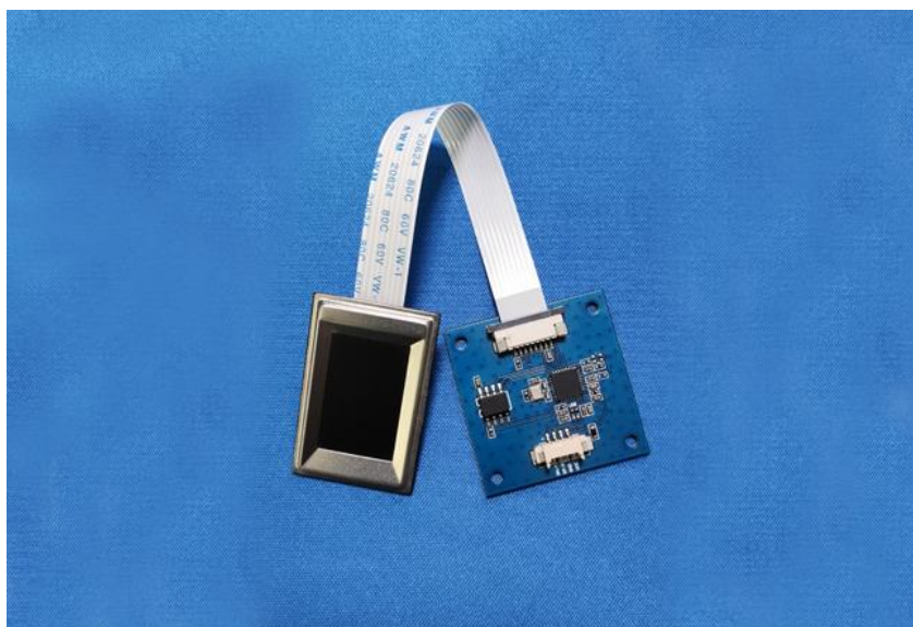
图2-1 GS25尺寸图
