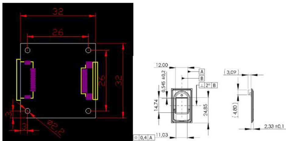
图2-1 S20尺寸图(正面兼容FPC1011结构，背面要空出两侧2mm用于固定)
