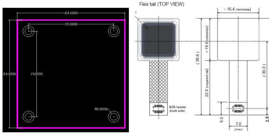
图2-1 S22尺寸图(正面兼容FPC1011结构, 背面要空出两侧2mm用于固定)
